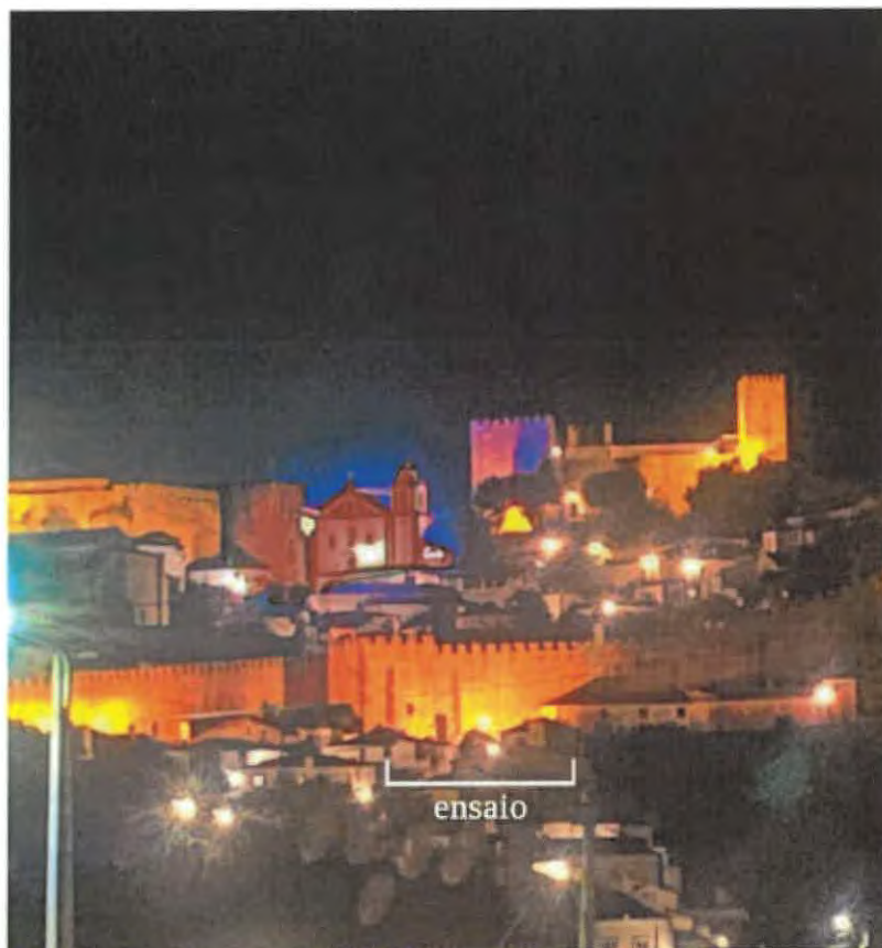
Ensaio realizado - no troço assinalado pode-se observar a iluminação ensaiada com LED 2200K, permitindo uma comparação directa com a restante iluminação em Sódio Alta Pressão
